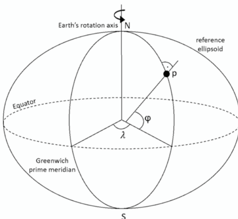
Фиг. 1.1.1.1. Схема на географска координатна система. Географските координати на точка p се определят от ъглите \phi (широчина) и \lambda (дължина)
